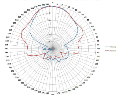
Diagrama de Radiación Antena 4GNOVA (2.2 GHz)
