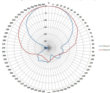
Diagrama de Radiación Antena 4GNOVA (800 MHz)
